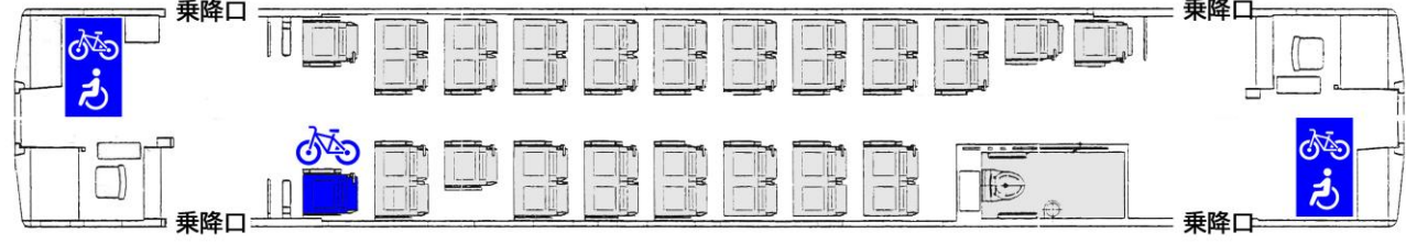
HSOR-150A形 最大3台（転換クロスシート1台、車いすスペース2台）
