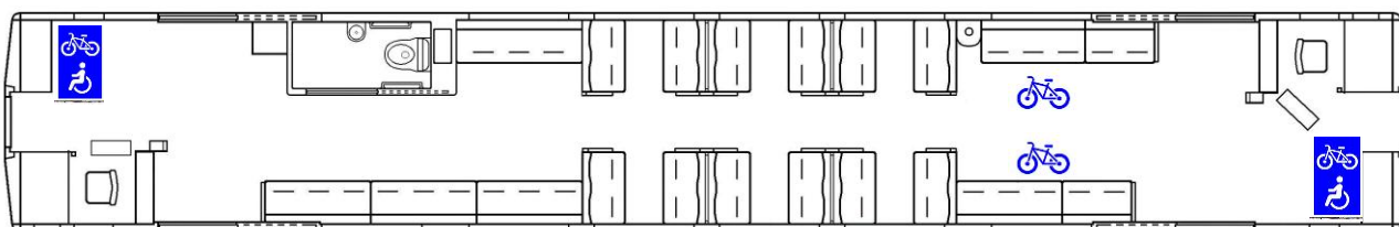
■ HSOR-100A形（上り列車：最大4台 下り列車：最大2台）
